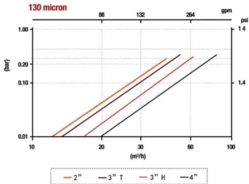
Perdidas de carga filtros disco retrolavado automático (120 Mesh)
