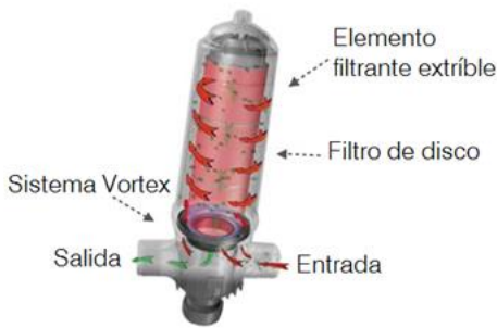
Esquema de funcionamiento modelo F90TDZ
