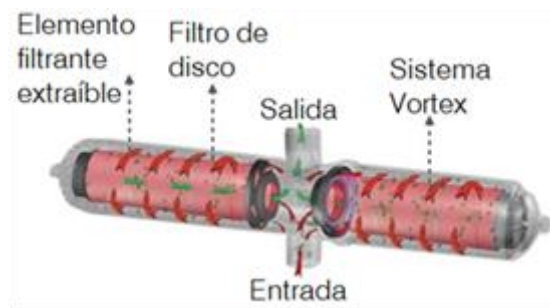
Esquema de funcionamiento modelo F110HDZ
