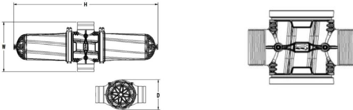
Esquema de dimensiones y conexión de modelo F110HDZ
