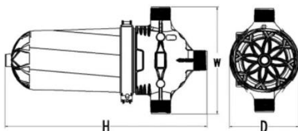
Esquema de dimensiones y conexión modelo F90TDZ
